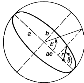
Рис. 55. Геометрические характеристики эллиптической траектории, истинная и эксцентриская аномалии
