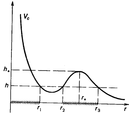
Рис. 51. Приведенный потенциал и зоны допустимых значений полярного радиуса
