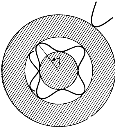
Рис. 50. Центральное поле сил и полярные координаты
