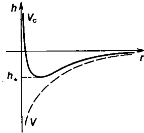
Рис. 53. Потенциал и приведенный потенциал в задаче Кеплера
